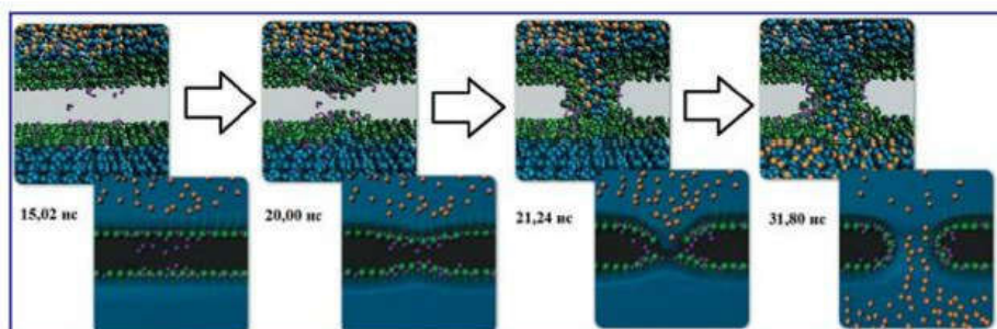
Рис. Образование пор в липидном бислое мембран клеток кожи после нанесения 10 мол.% ДМСО. Вода обозначена синим цветом, ДМСО фиолетовым, группы липидных головок зеленым, препарат желтым [25]
